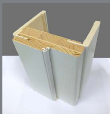
Telaio Listellare BT44 coprifili 70/90 in multistrato
