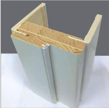
Telaio piatto listellare Coprifilo piatto multistrato 70/90 mm
