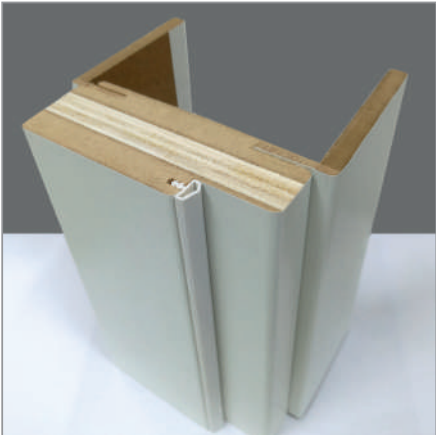
Telaio piatto Sandwich Coprifilo piatto MDF da 70 mm
